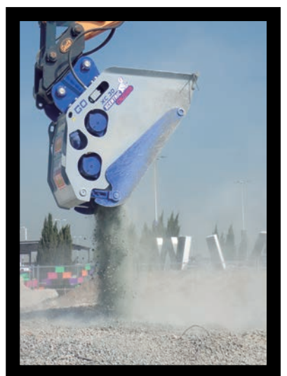
Xcentric Crusher en démonstration sur l'espace Pole Mat.
